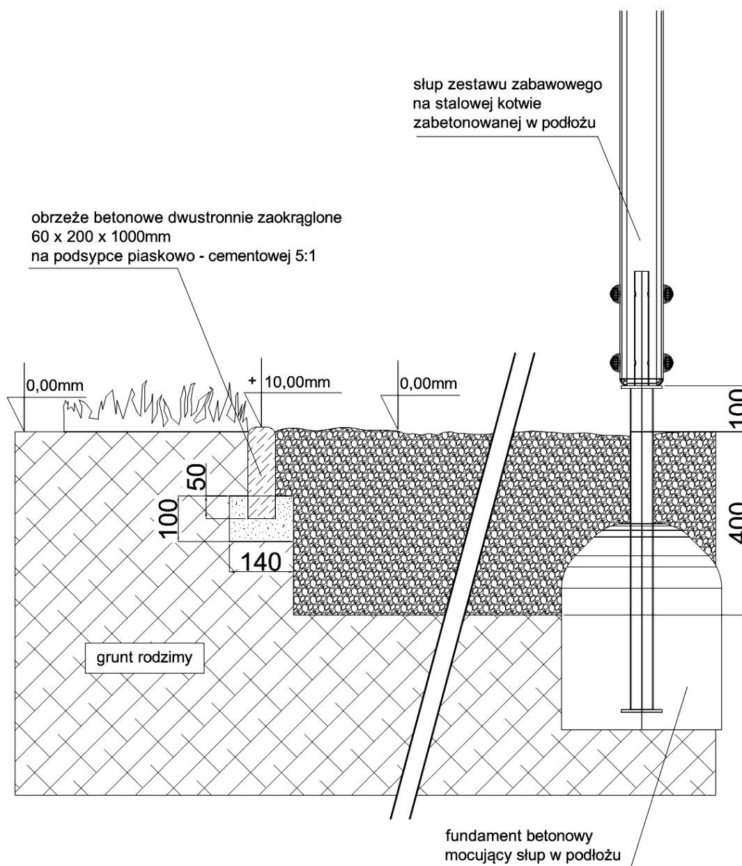
Rys. 17 Przekrój przez pole żwirowe A oraz posadzenie słupa w podłożu. (W przypadku pola żwirowego B warstwa żwirku / głębokość wykopu 300mm).
