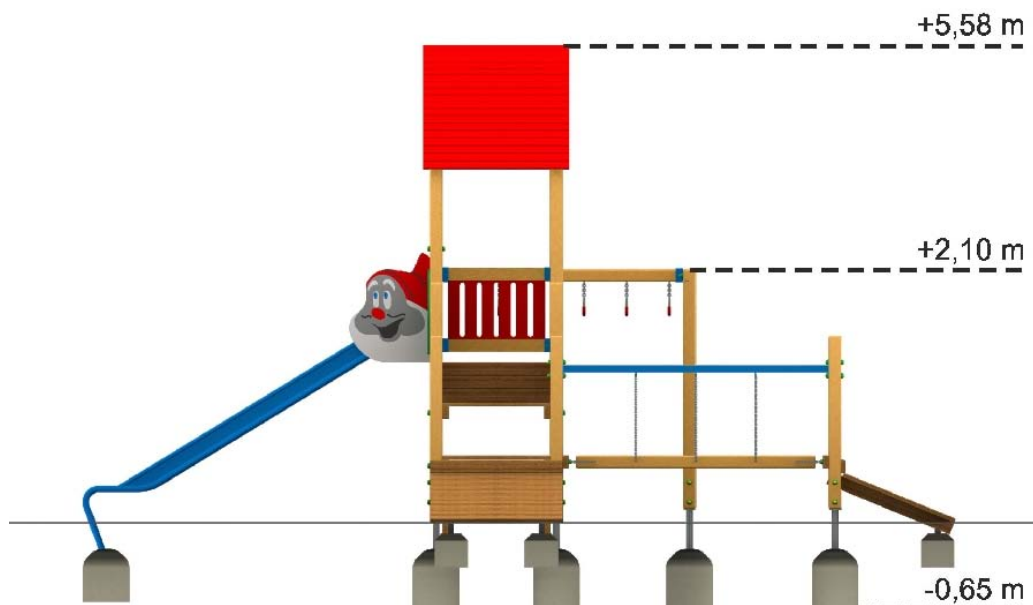
Rys. 2 Zestaw zabawowy – ogólnorozwojowy typu Mędrak-5 (widok z boku).
