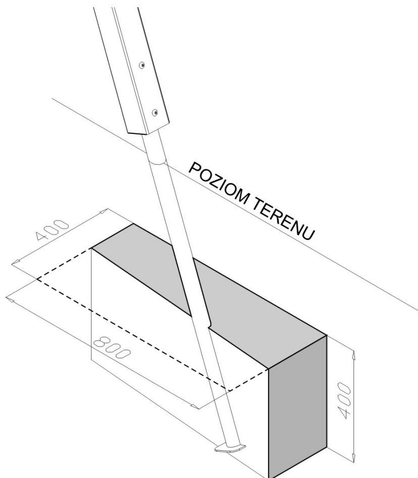
Rys. 16 Schemat fundamencie słupa skośnego (na przykładzie nogi / słupa huśtawki wahadłowej).
